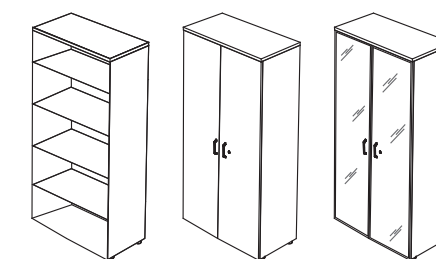
90x45x196h
