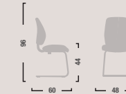
QD25 Sedia fissa senza braccioli. Fixed chair.
